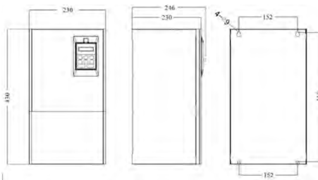
Рис. 1-7. Габаритные размеры преобразователей частоты с мощностью от 30 кВт до 37 кВт
